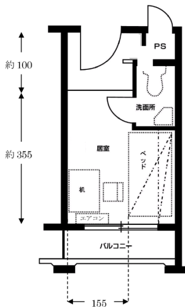
(居室平面図)
