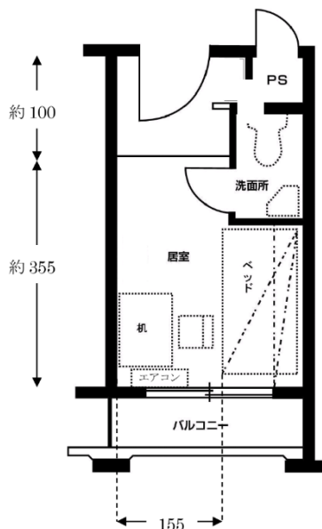
(居室平面図)
