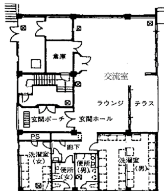
(1 階)
